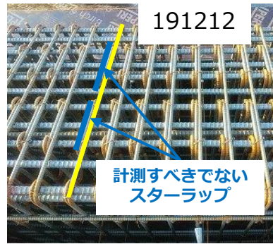
スターラップで2本分を計測
